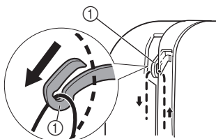
① Fadenhebel
