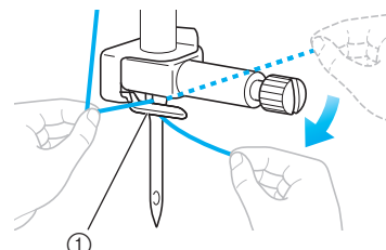
① Fadenführung der Nadelstange
