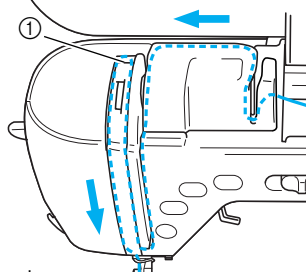
① Verriegelung
