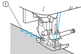
① Nadeleinstichpunkt
