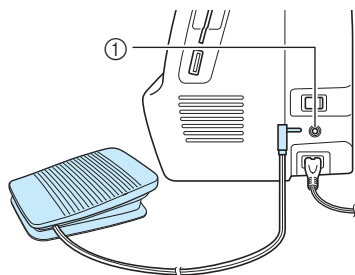
① Fußpedal-Anschlussbuchse
