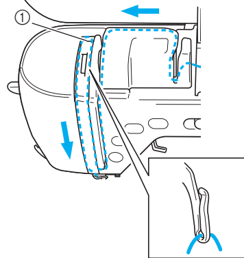
① Verriegelung
