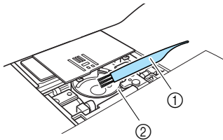
① Reinigungspinsel ② Greifergehäuse
