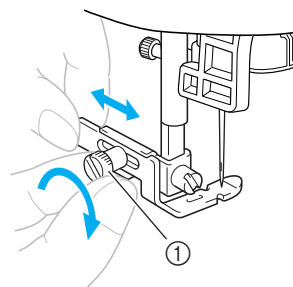
① Fixierschraube
