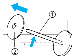
① Garnrollenstift ② Garnrollenkappe
