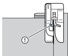
① Nadeleinstichpunkt
