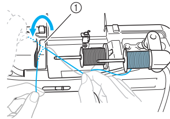
① Fadenführungsdeckel
