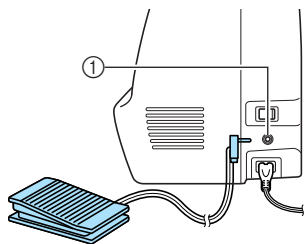
① Fußpedal-Anschlussbuchse
