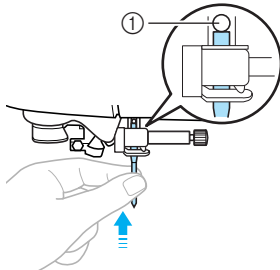
① Nadelanschlag
