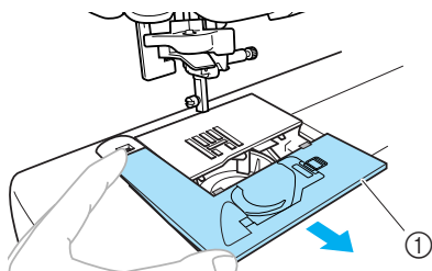
① Stichplattenabdeckung
