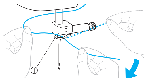
① Fadenführung der Nadelstange
