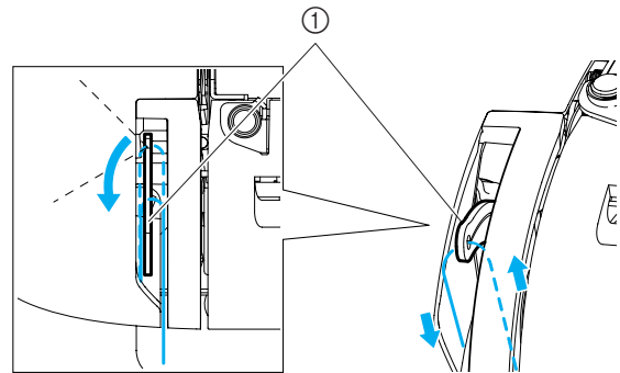
① Fadenhebel
