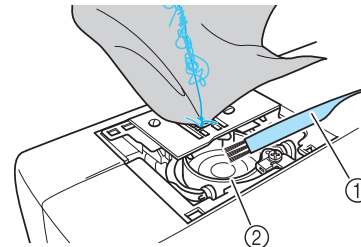
① Reinigungspinsel ② Greifergehäuse
