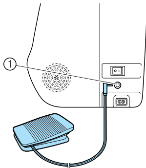
① Fußpedal-Anschlussbuchse
