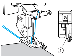
① Führung
