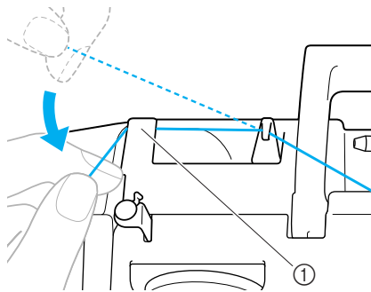
① Fadenführungsdeckel
