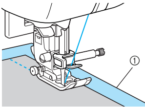
① Stickunterlegvlies oder Papier
