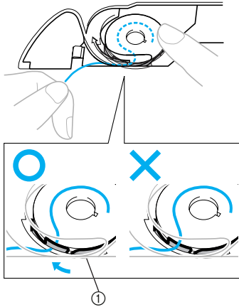
① Spannungseinstellfeder
