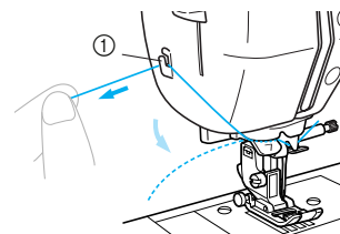
① Fadenabschneider
