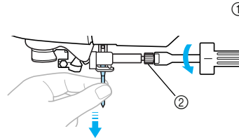
① Schraubendreher ② Nadelklemmschraube
